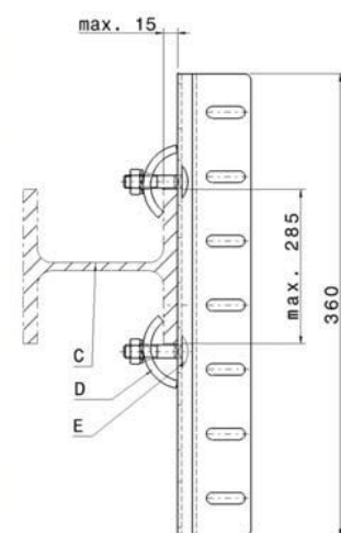
C: 梁直立
