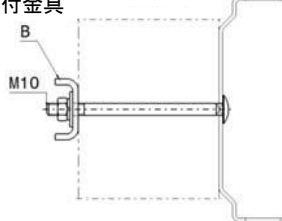
X 矢視図
