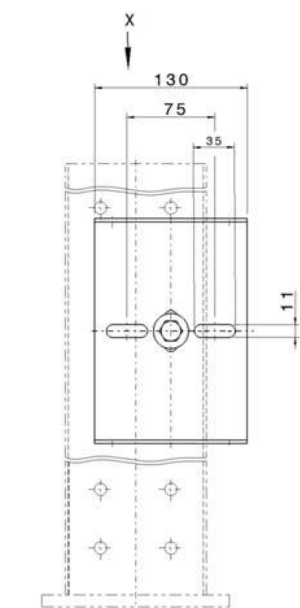
X 矢視図
