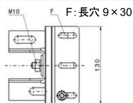
F: 長穴 9×30
