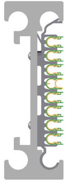
U10 コンダクターレール (3 相+PE-VPN+4 極) を含むコンパクトハンガー
