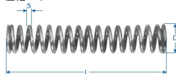
圧縮バネ DF
