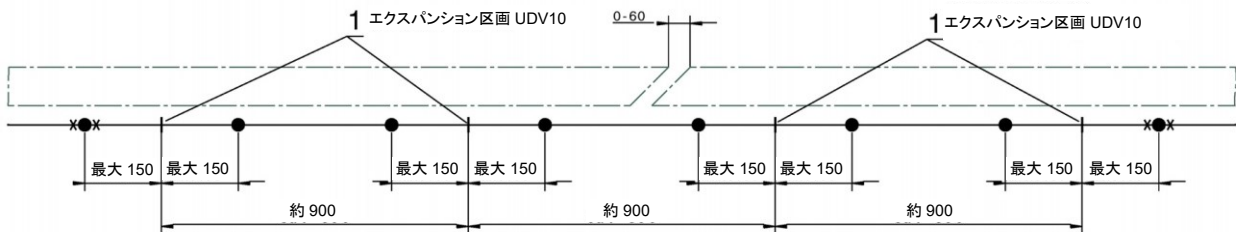
図 6-4: エクspansion区画 UDV10/C-60、伸縮寸法最大 60mm。
