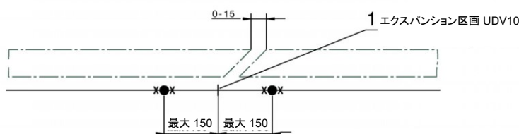
図 6-1: エクspansion区画 UDV10/C-15、伸縮寸法最大 15mm。
