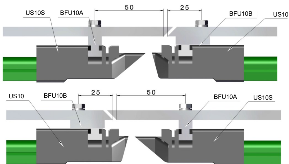
特殊保護接地(PE-VPN)用、ストレート、システム取付高さ 16.5mm
