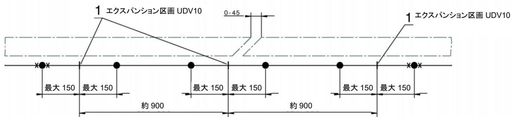
図 6-3: エクspansion区画 UDV10/C-45、伸縮寸法最大 45mm。
