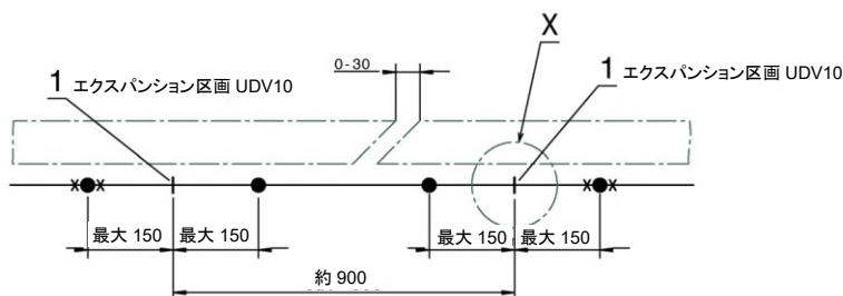
図 6-2: エクspansion区画 UDV10/C-30、伸縮寸法最大 30mm。
