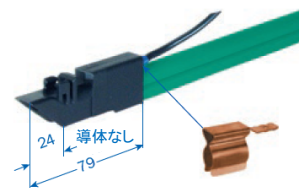
給電クリップ付: USE10S (斜め) (平形端子 6.3 × 0.8mm 用)
