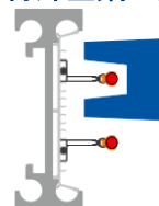
EMS 特殊型鋼に設置
