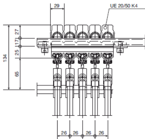
配置図
