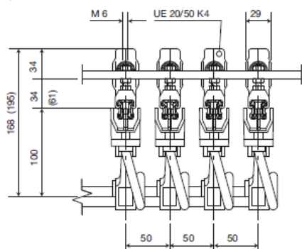
配置図
