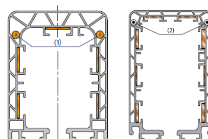
(1) KBH (2) MKH ヒータィングケーブル配置(両側)
