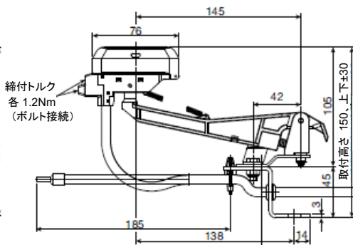
KESL組立図
