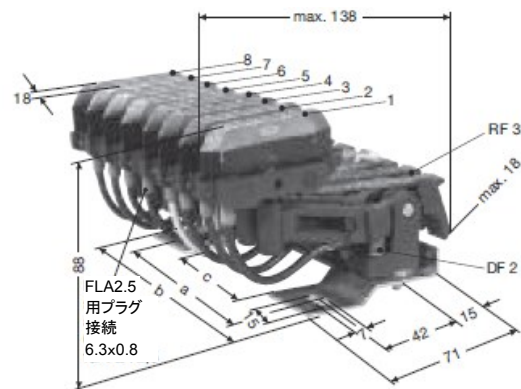
KESL組立図
