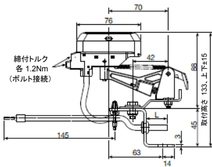
KESR組立図
