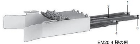
EM20 4極の例
