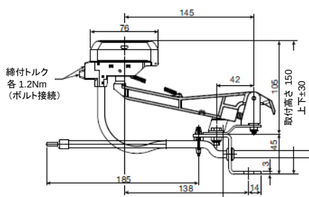
KESL組立図
