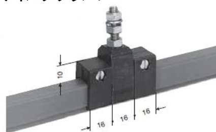
絶縁ハンガーとロケーティングクランプ2個使用(固定点)
