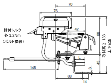
KESR組立図
